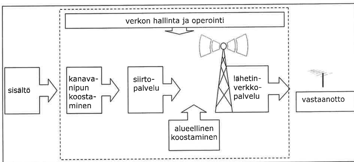
Kuva 1. Digitaalisen televisiölähetyksetverkon perusrakenne
