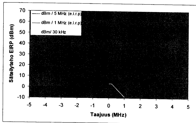
Kuva 2. Taajuuskaistan ulkopuoliset läheteet 0-5 MHz päähän taajuuskaistan yläreunasta.
